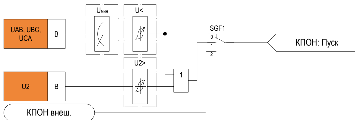
Рисунок 2.2 – Функциональная схема «КПОН»
