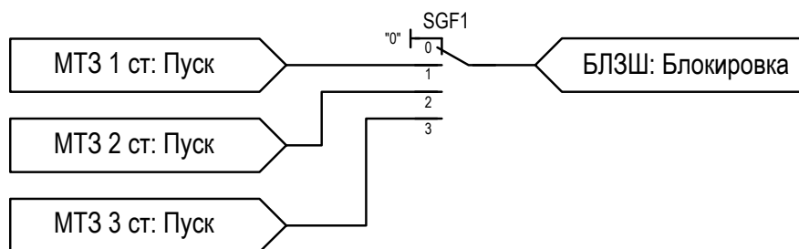
Рисунок 2.4 – Функциональная схема БЛЗШ
